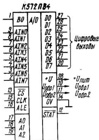
Типовая схема включения ИС К572ПВ4
