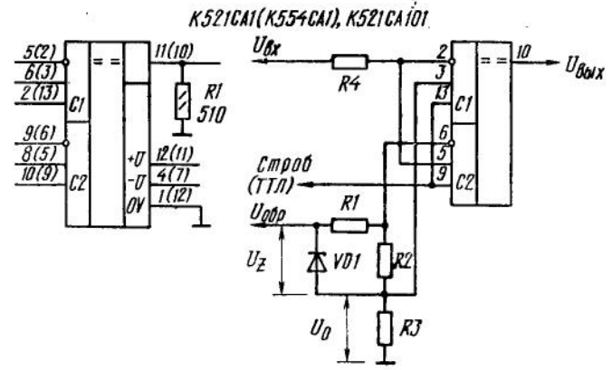
Типовая схема включения ИС K521(554)CA1, K521CA101
