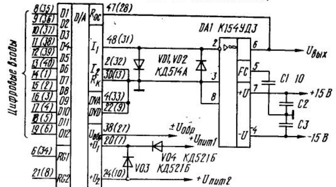
Типовая схема включения ИС К(Р)572ПА2А (Б, В)
