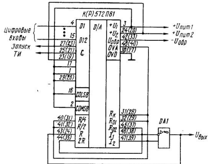
Схема включения ИС (КР)572ПВ1А(Б, В) в режиме ЦАП с параллельным входом
