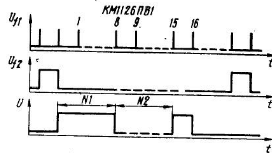
Временные диаграммы работы ИС КМ1126ПВ1
