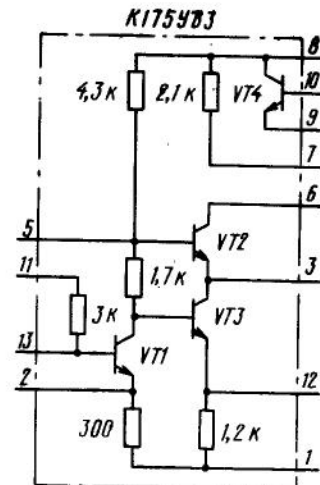
Принципиальная схема ИС К175УВ3А (Б)
