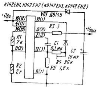
Схема включения ИС К(Р)142ЕН1А (Б—Г), К(Р)142ЕН2А (Б—Г) для улучшения коэффициентов K_{нУИ} K_{нI}
