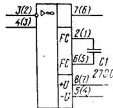
Типовая схема включения ОУ К(Р)574УД3
