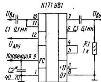
Типовая схема включения ИС К171УВ1
