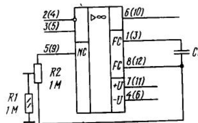
Типовая схема включения ОУ К153(553)УД2, К553УД201, К740УД5-1
