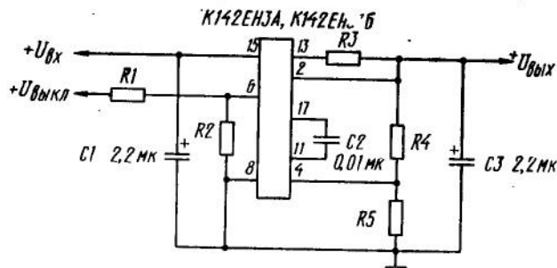
Типовая схема включения ИС K142EN3A (Б), K142EN4A (Б)
