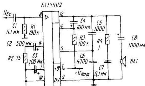
Типовая схема включения ИС К174УН9А(Б)
