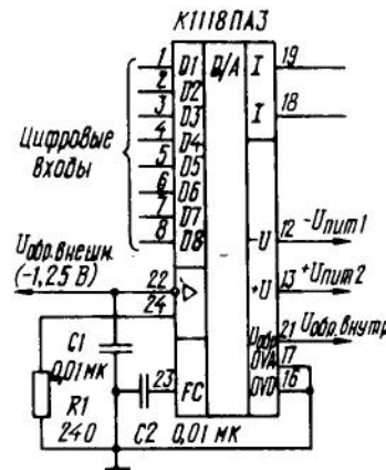
Типовая схема включения ИС К1118ПАЗ. Прямой аналоговый выход — вывод 18, инверсный — 19.
