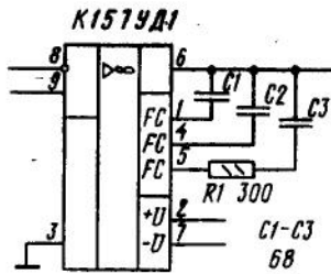
Типовая схема включения ОУ К157УД1
