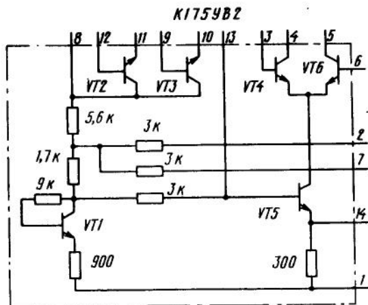
Принципиальная схема ИС К175УВ2А (Б)
