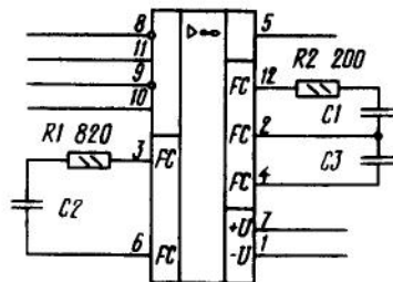
Типовая схема включения ОУ К140УД5А(Б)
