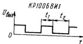
Временная диаграмма выходного сигнала мультвибратора
