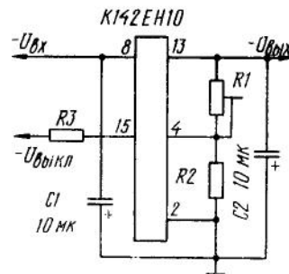
Типовая схема включения ИС К142ЕН10
