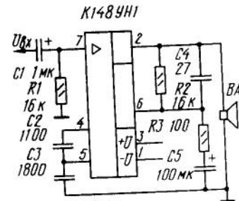
Типовая схема включения ИС К148УН1
