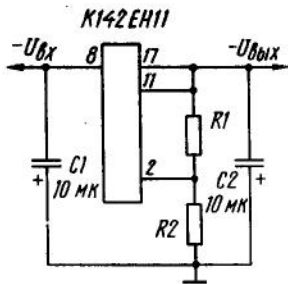
Типовая схема включения ИС К142ЕН11
