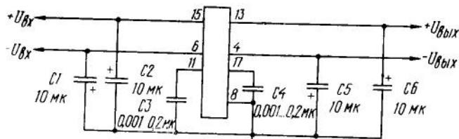
Типовая схема включения ИС К142ЕН6А (Б—Г) К142ЕН6А — К142ЕН6Г
