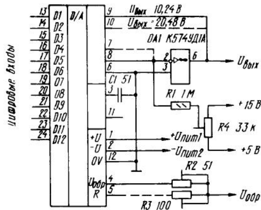
Типовая схема включения ИС К1108ПА1А (Б)
