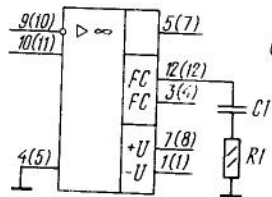
Типовая схема включения ОУ К(P)140УД1А(Б)
