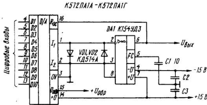
Типовая схема включения ИС К572ПА1А (Б-Г)
