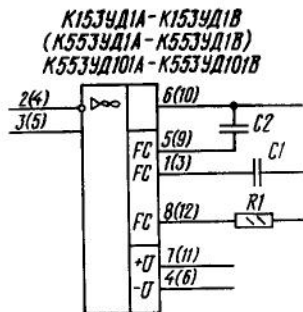
Типовая схема включения ОУ К153(553)УД1А (Б, В), К553УД101А (Б, В)
