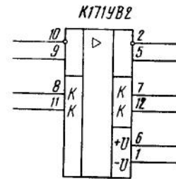
Типовая схема включения ИС К171УВ2
