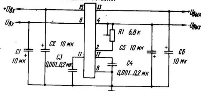
Схема включения ИС К142ЕН6А (Б—Г) для получения стабилизированного напряжения от 2 \times 15 до 2 \times 27 В
