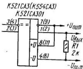
Схема включения ИС К521(554)СА3 с эмиттерным выходом
