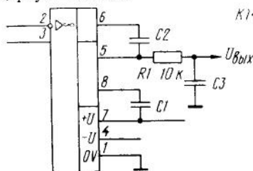
Типовая схема включения ОУ K140УД13
