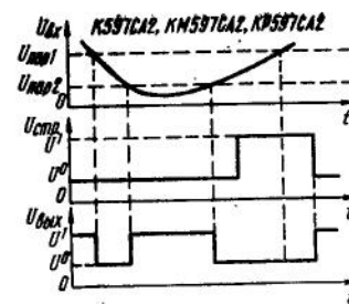
Временные диаграммы работы детектора-ограничителя по двум уровням на ИС К(М, Р)597СА2
