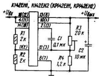
Схема включения ИС К(Р)142ЕН1А (Б—Г), К(Р)142ЕН2А (Б—Г) для увеличения быстродействия защиты от короткого замыкания и в нагрузке
