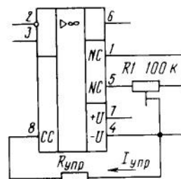
Типовая схема включения ОУ К140УД12, КР140УД1208
