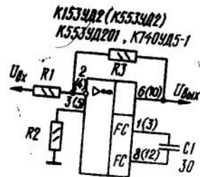
Схема включения ОУ К153(553)УД2, К553УД201, К740УД5-1 со стандартной частотной коррекцией
