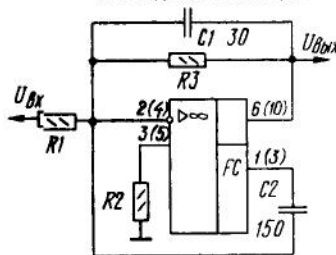
Схема включения ОУ К153(553)УД2, К553УД201, К740УД5-1 с частотной коррекцией с опережением по ВЧ составляющим
