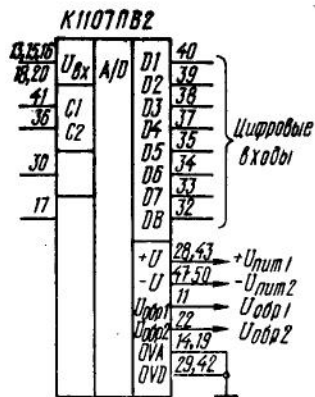
Типовая схема включения ИС К1107PB2
