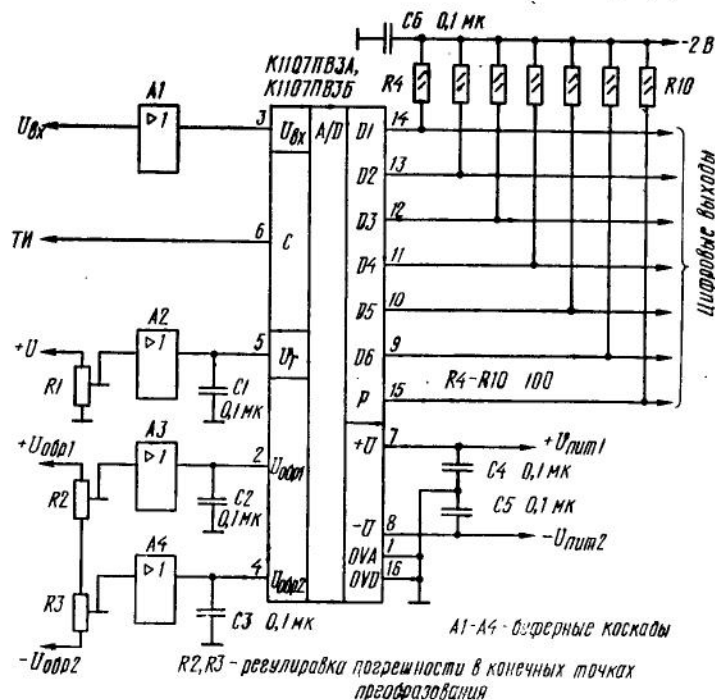
Типовая схема включения ИС К1107PB3A (Б)
