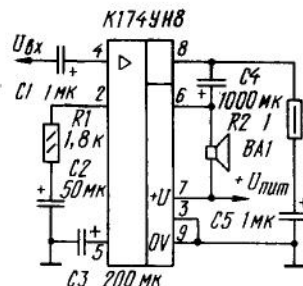
Типовая схема включения ИС К174УН8
