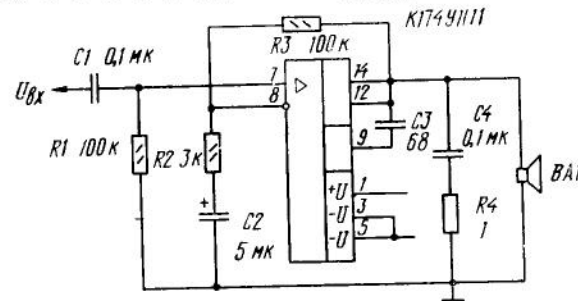
Типовая схема включения ИС К174УН11
