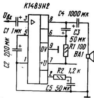
Типовая схема включения ИС К148УН2
