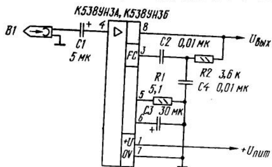
Типовая схема включения ИС К538УН3А (Б)
