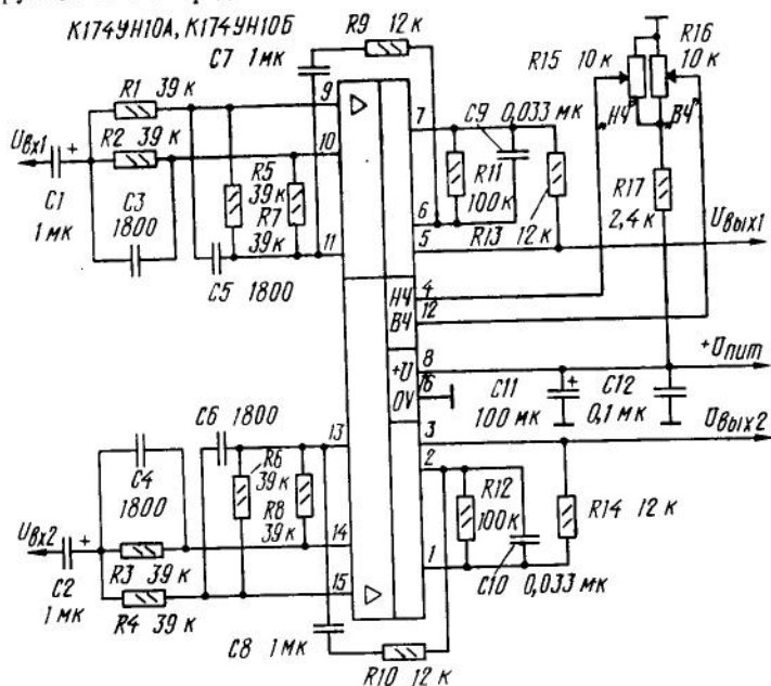
Типовая схема включения ИС К174УН10А (Б)
