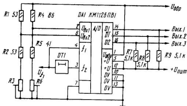
Типовая схема включения ИС КМ1126ПВ1
