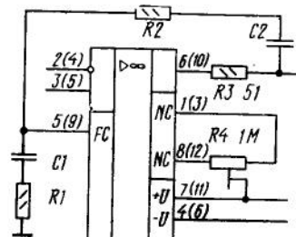
Типовая схема включения ОУ К(Р, М)551УД1А (Б)
