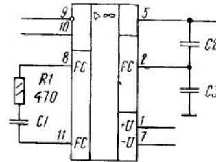
Типовая схема включения ОУ К140УД2А(Б)
