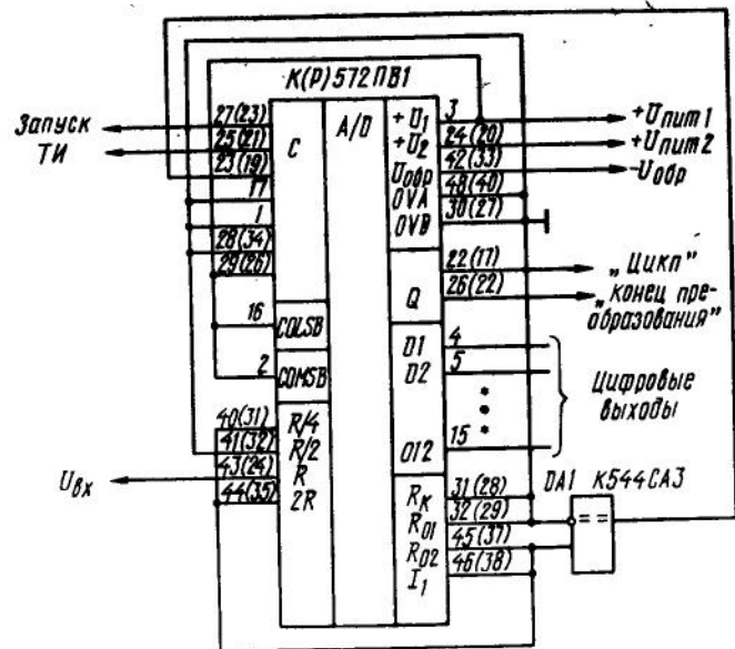
Схема включения ИС К(Р)572ПВ1А (Б, В), обеспечивающая максимальное быстродействие
