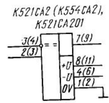
Типовая схема включения ИС K521(554)CA2, K521CA201
