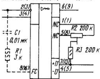
Типовая схема включения ОУ К(Р)140УД11, КР140УД1101
