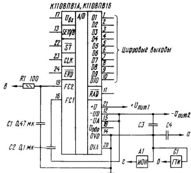
Типовая схема включения ИС К1108PB1А (Б)
