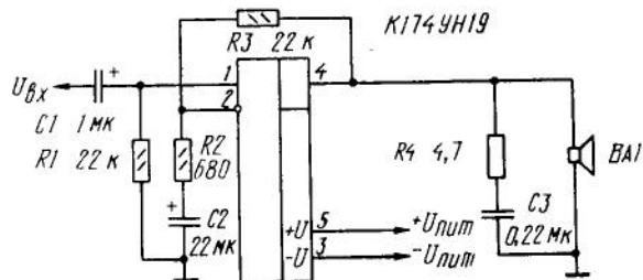
Типовая схема включения ИС К174УН19
