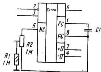
Типовая схема включения ОУ К153УД6
