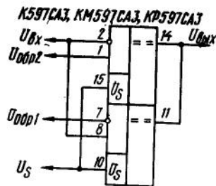
Принципиальная схема детектора погодовых уровней на ИС К(М, Р)597СА3
