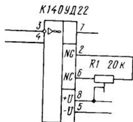
Типовая схема включения ОУ К140УД22
