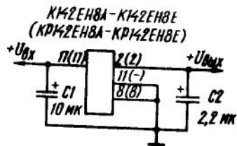
Типовая схема включения ИС К(Р)142ЕН8А (Б-Е)
