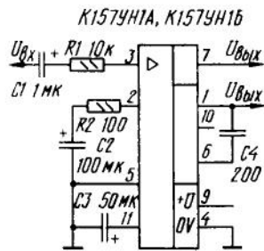
Типовая схема включения ИС К157УН1А (Б)
