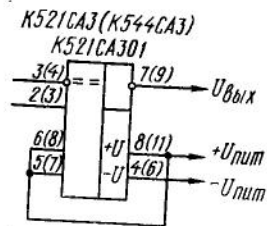
Схема включения ИС К521(554)СА3 для увеличения быстродействия
