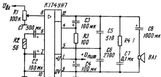
Типовая схема включения ИС К174УН7
