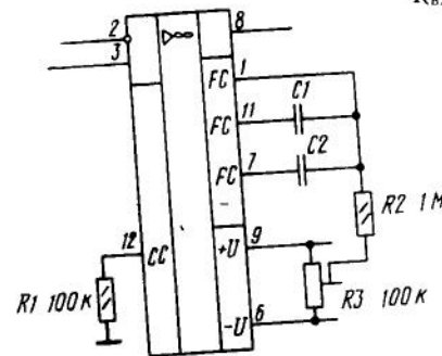
Типовая схема включения ОУ K153UD4
