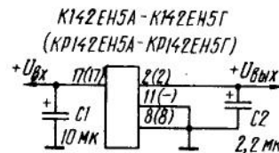
Типовая схема включения ИС K(P)142EN5A (Б-Г)
