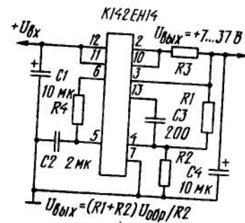
Схема включения ИС К142ЕН14 для получения стабилизированного напряжения от 7 до 37 В
