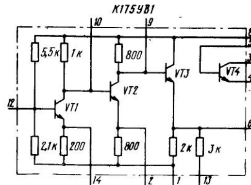
Принципиальная схема ИС К175УВ1А(Б)
