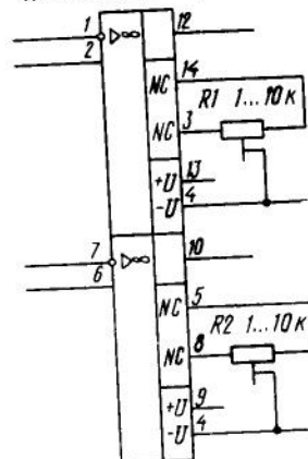
Типовая схема включения ОУ К(Р)140УД20
