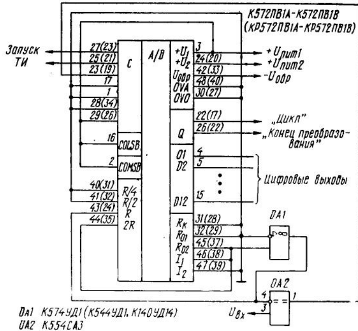
Схема включения ИС К(Р)572ПВ1А (Б, В), обеспечивающая максимальную точность и стабильность преобразования
