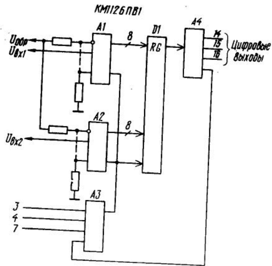
Структурная схема ИС КМ1126ПВ1
