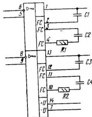
Типовая схема включения ОУ К(Р)551УД2А (Б)
