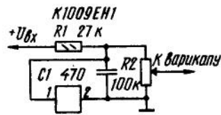
Типовая схема включения ИС К1009ЕН1
