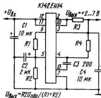
Схема включения ИС К142ЕН14 для получения стабилизированного напряжения от 2 до 7 В
