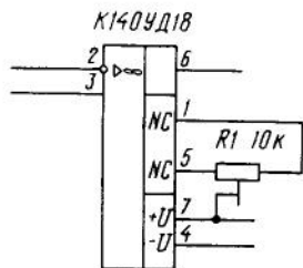
Типовая схема включения ОУ К140УД18
