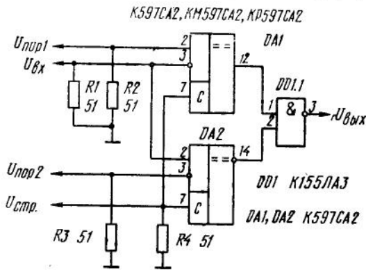
Принципиальная схема детектора-ограничителя по двум уровням с запоминанием на ИС К(М, Р)597СА2
