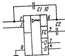
Типовая схема включения ОУ К154УД4А(Б)
