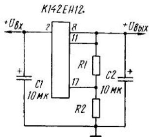
Типовая схема включения ИС К142ЕН12
