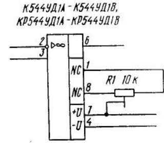
Типовая схема включения ОУ К(Р)544УД1А (Б, В)
