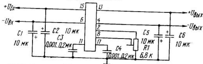
Схема включения ИС К142ЕН6А (Б—Г) для получения стабилизированного напряжения от 2 \times 4,5 до 2 \times 15 В
