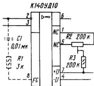
Типовая схема включения ОУ К140УД10
