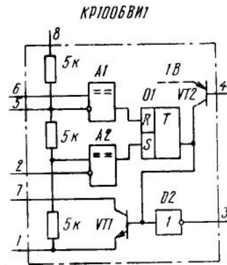
Структурная схема таймера КР1006ВИ1
